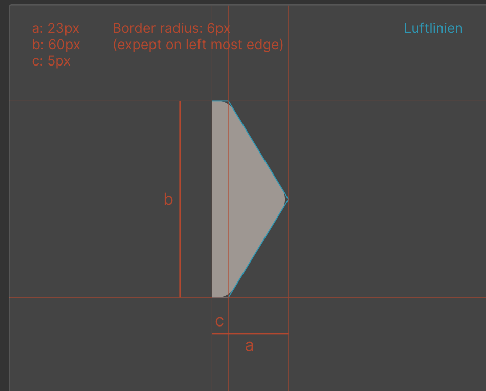
Figma Komponente
